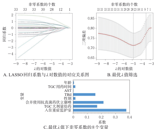
图1 LASSO 回归分析筛选非零系数预测变量的过程
