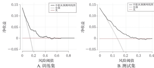
图5 列线图预测模型的DCA结果
