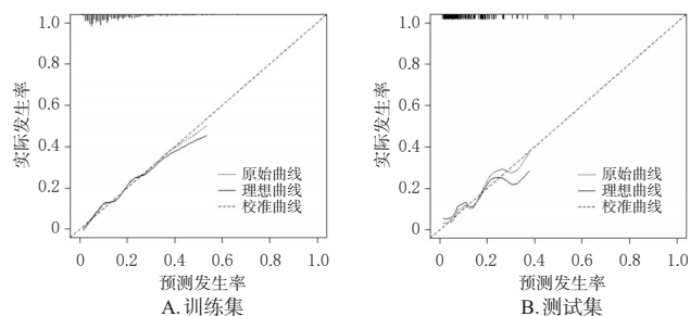
图4 列线图预测模型的校准曲线
