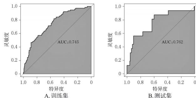
图3 列线图预测模型的ROC曲线分析
