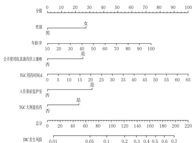
图2 TGC相关DIC预测模型的列线图
